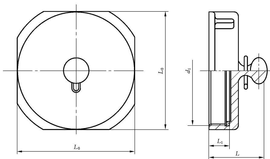
图 2 KA 型阀盖
