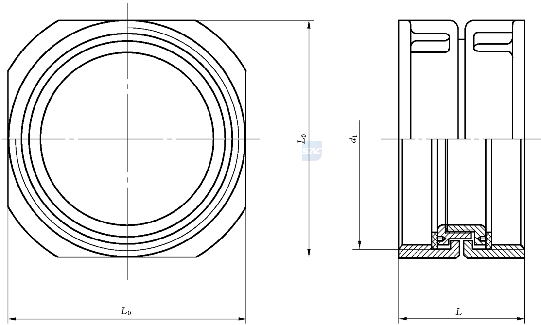
图 3 KT 型同型接口
