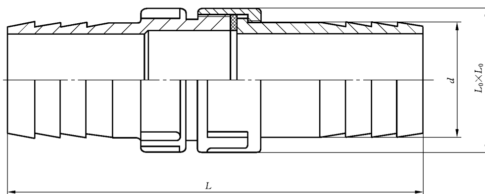
a) 总图
