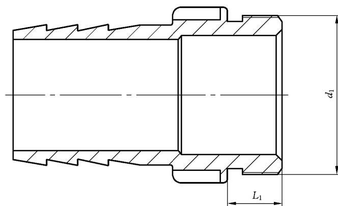
b) 雄接头
