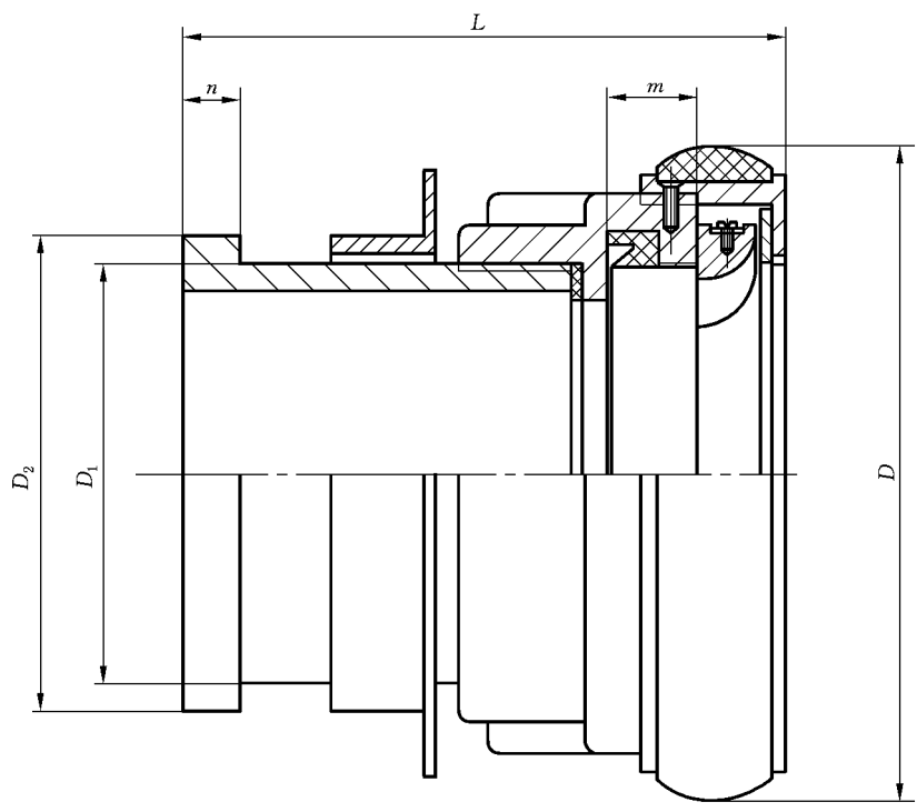
图 4 KJK 型异径接口
