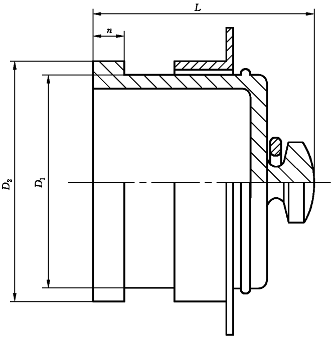
图 5 KMK 型阀盖
