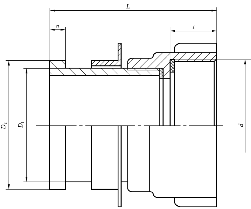
图 3 KYKA 型管牙雄接口
