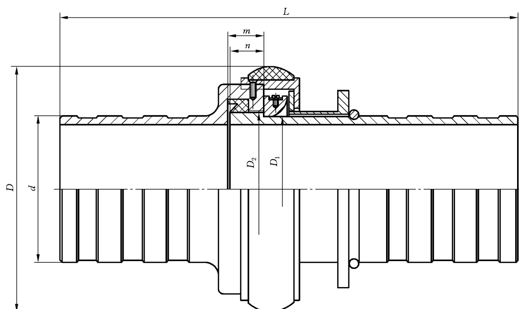
图 1 KDK 型水带接口
