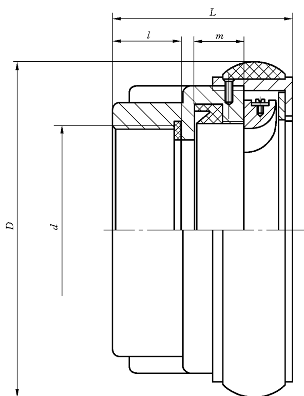
图 2 KYK 型管牙雌接口
