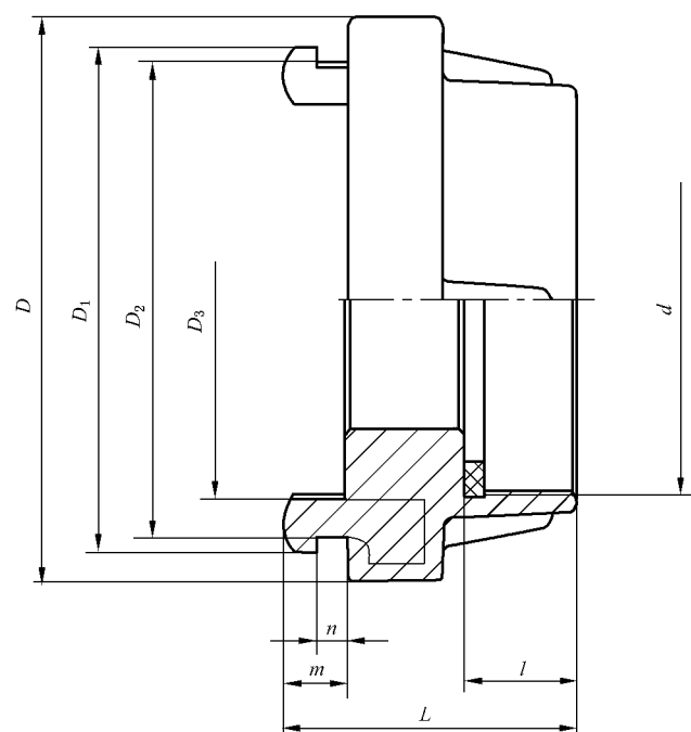
图 5 KN 型内螺纹固定接口
