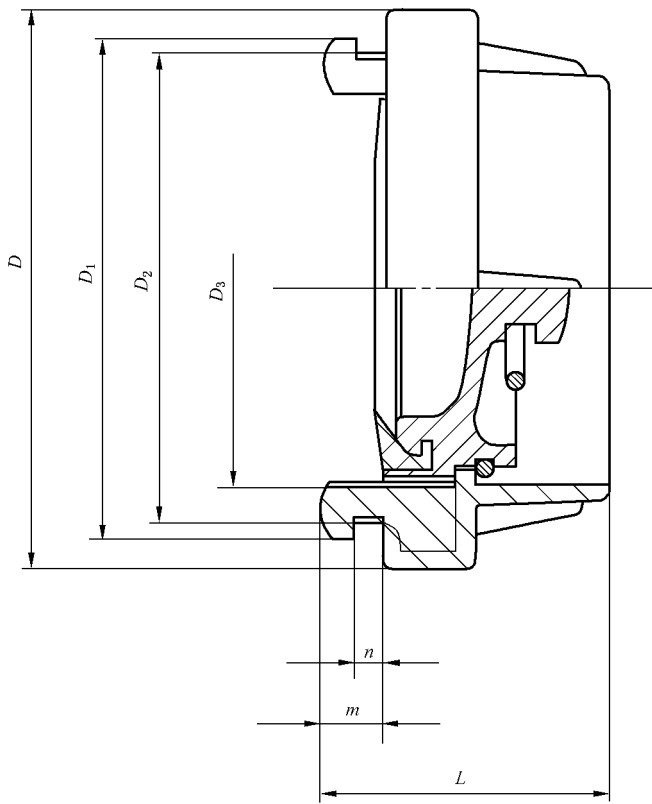
图 4 KM 型闷盖
