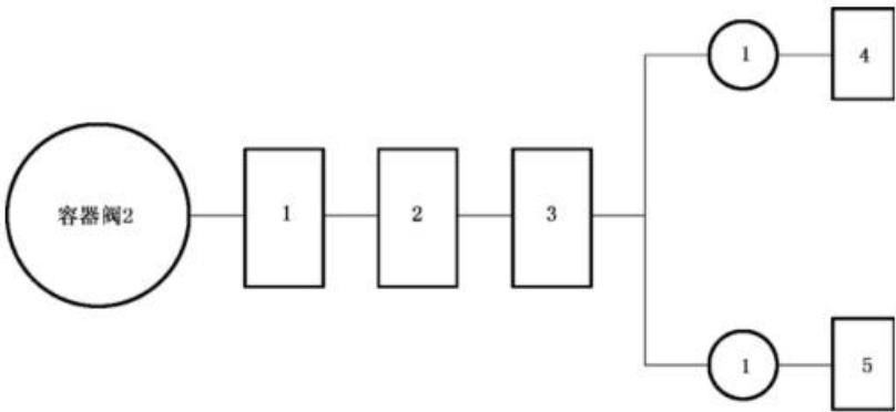
图 B.1 容器阀试验程序图
