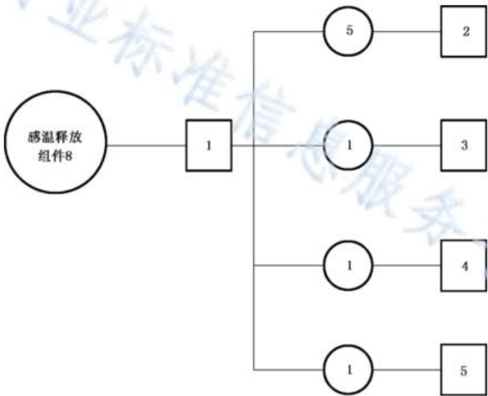
图 B.3 感温释放组件试验程序图
