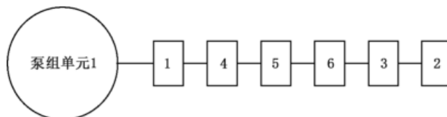
图 G.1 泵组单元试验程序图
