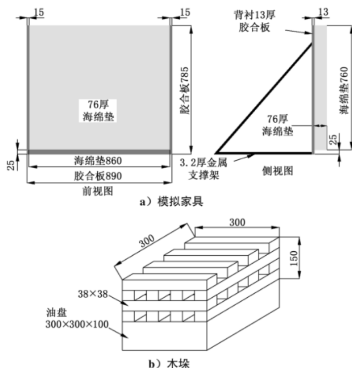
图6 木垛及模拟家具图
