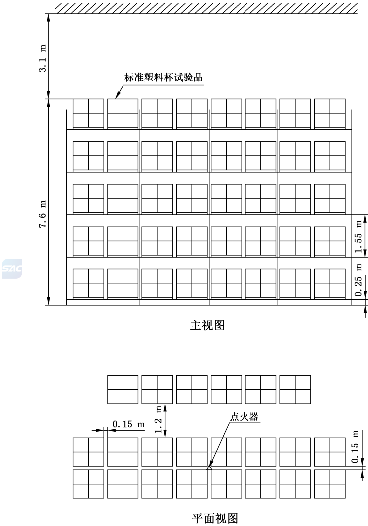
图 17 K 282 下垂型 CMSA 喷头灭火试验布置——试验 5
