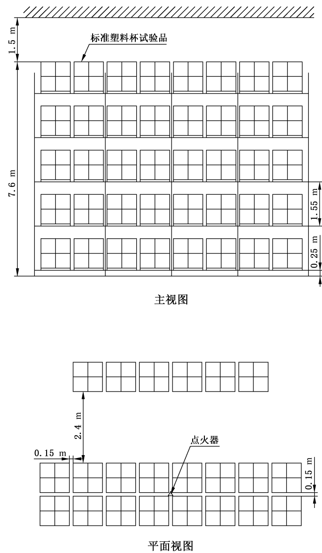
图 21 K 363 下垂型 CMSA 喷头灭火试验布置——试验 3
