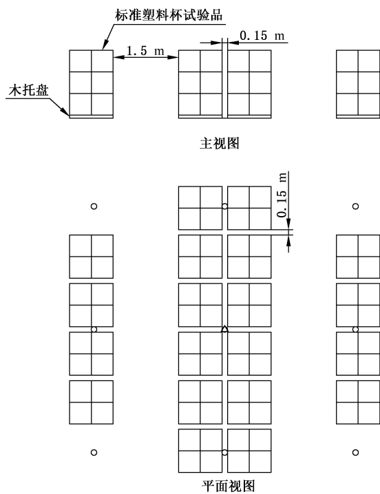
图6 标准纸杯试验品堆垛图（点火位置在1只喷头正下方）
