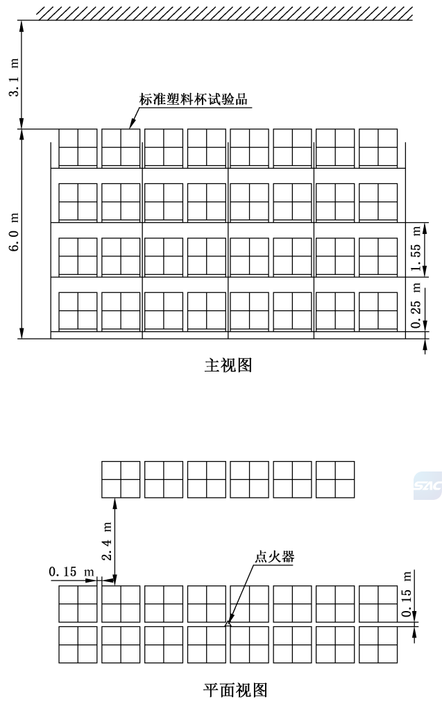
图 25 K 363 的直立型 CMSA 喷头灭火试验布置——试验 1
