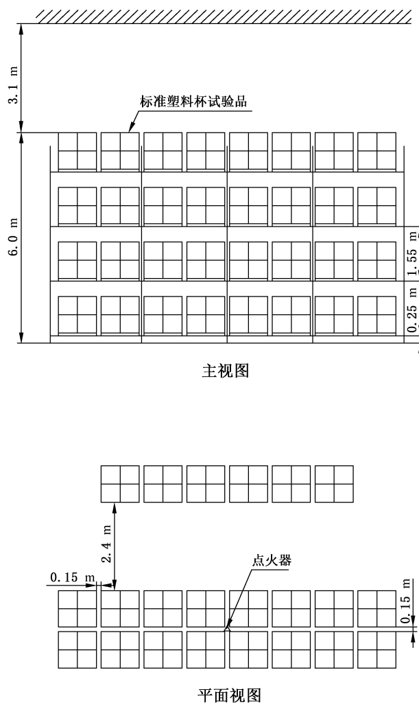
图 20 K 363 下垂型 CMSA 喷头灭火试验布置——试验 2
