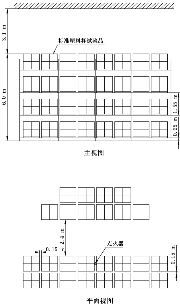
图 8 K 161 CMSA 喷头灭火试验布置——试验 1
