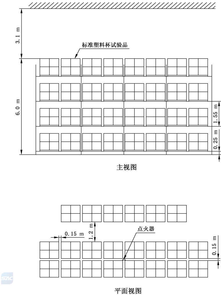
图 13 K 282 下垂型 CMSA 喷头灭火试验布置——试验 1
