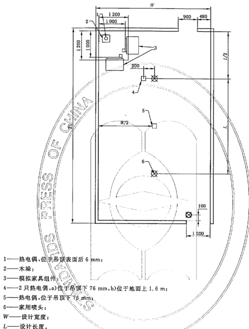
图 6 非边墙型喷头灭火试验布置图
