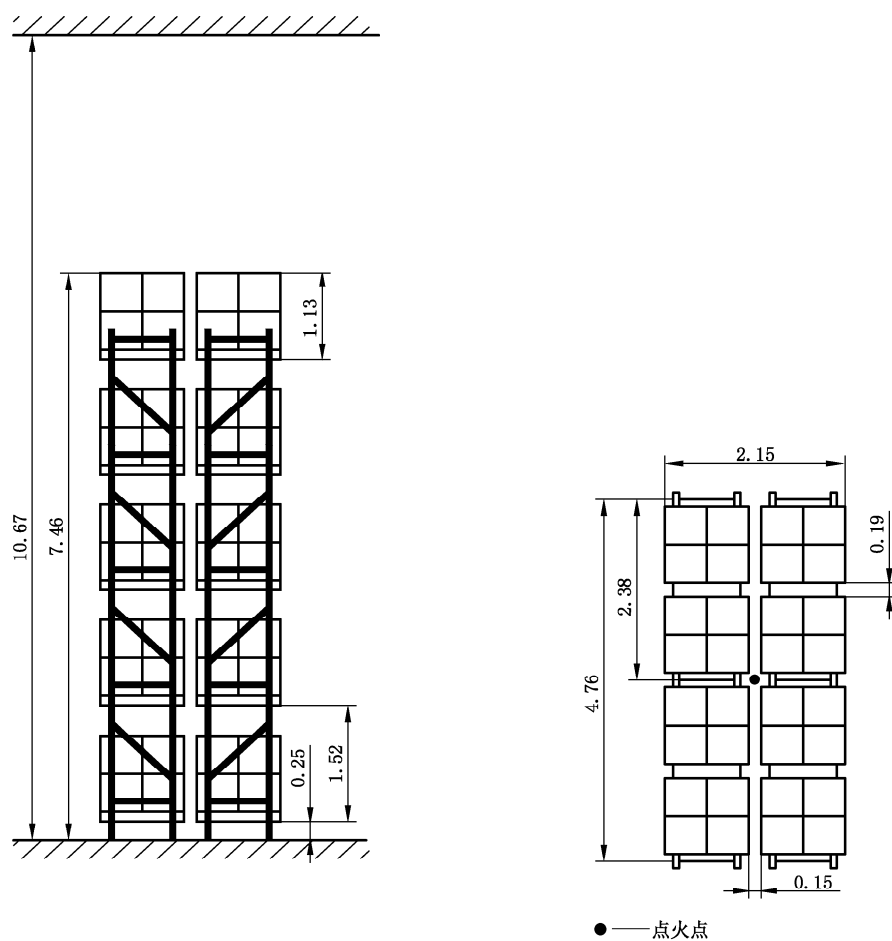
图 15 K 202 直立型 ESRF 喷头灭火试验布置 试验 D
