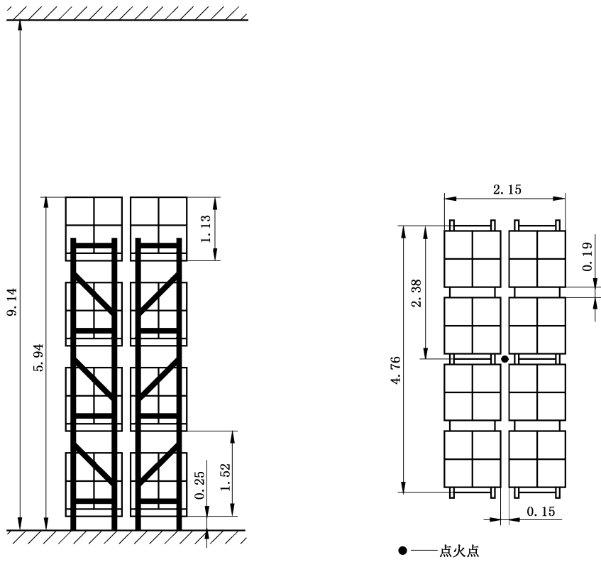
图 23 K 323 下垂型 ESFR 喷头灭火试验布置 试验 B
