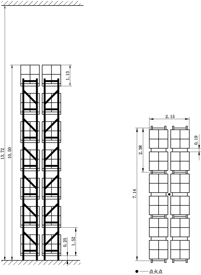
图 29 K 363 下垂型 ESFR 喷头灭火试验布置 试验 D
