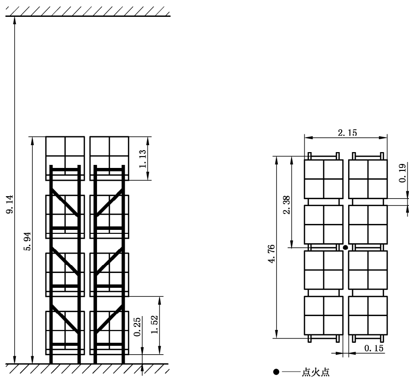
图 12 K 202 直立型 ESRF 喷头灭火试验布置 试验 A
