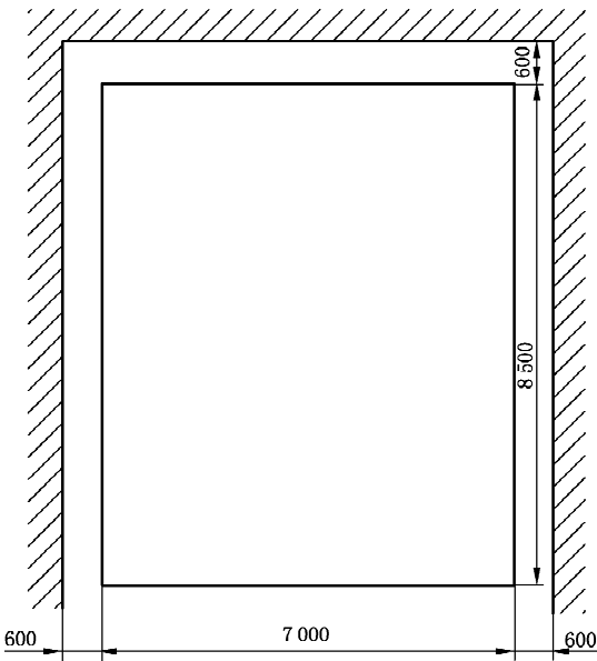
图 2 布水试验装置吊顶
