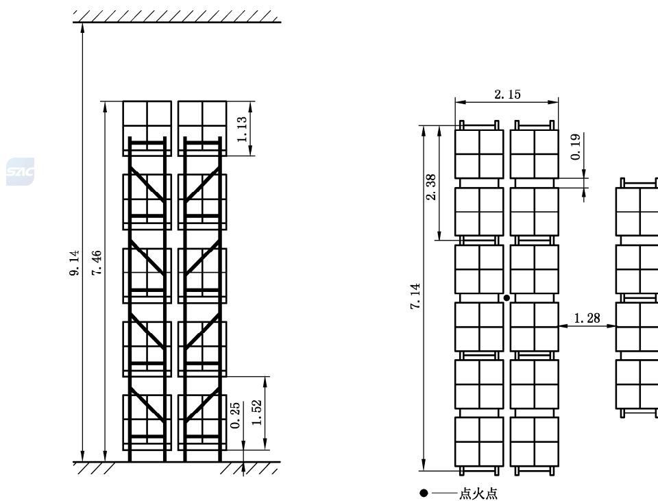
图 13 K 202 直立型 ESRF 喷头灭火试验布置 试验 B
