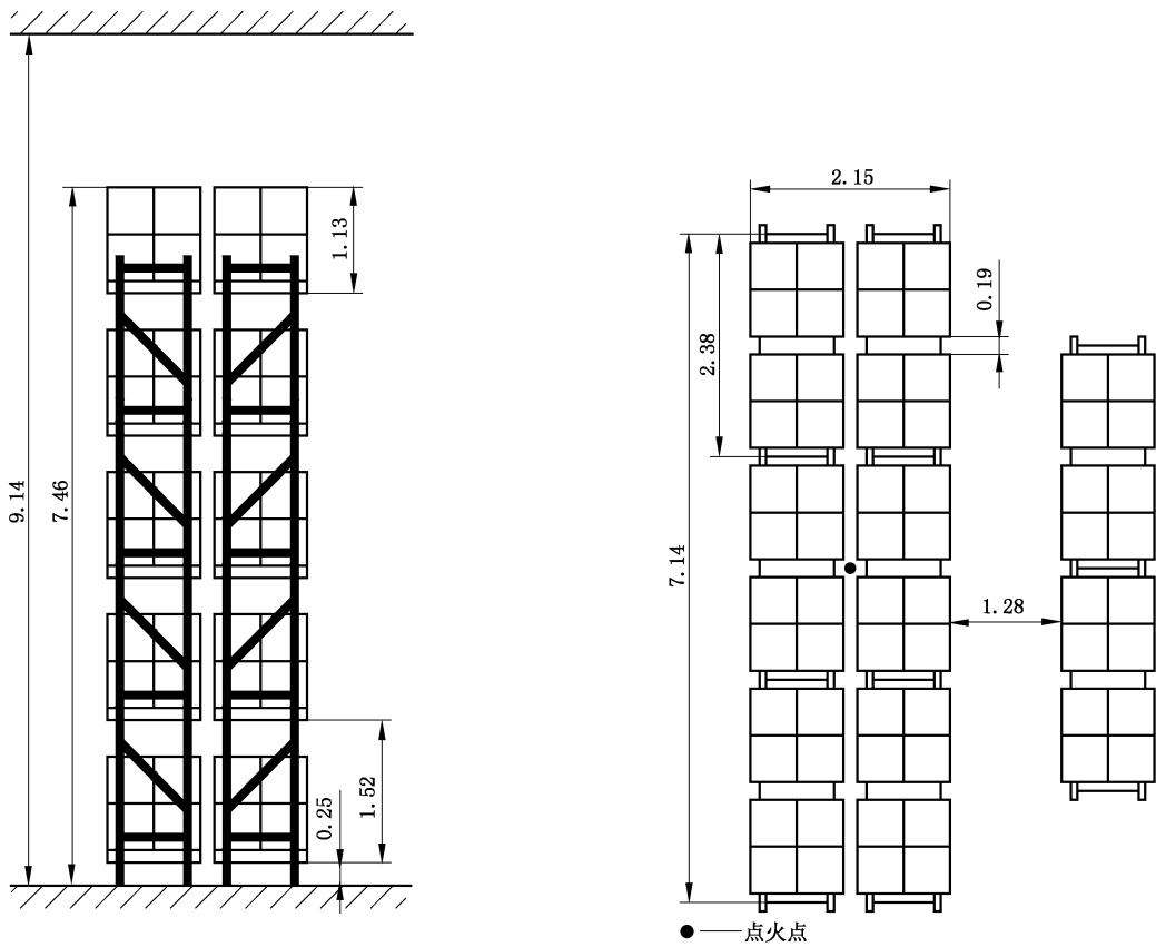
图 26 K 363 下垂型 ESRF 喷头灭火试验布置 试验 A
