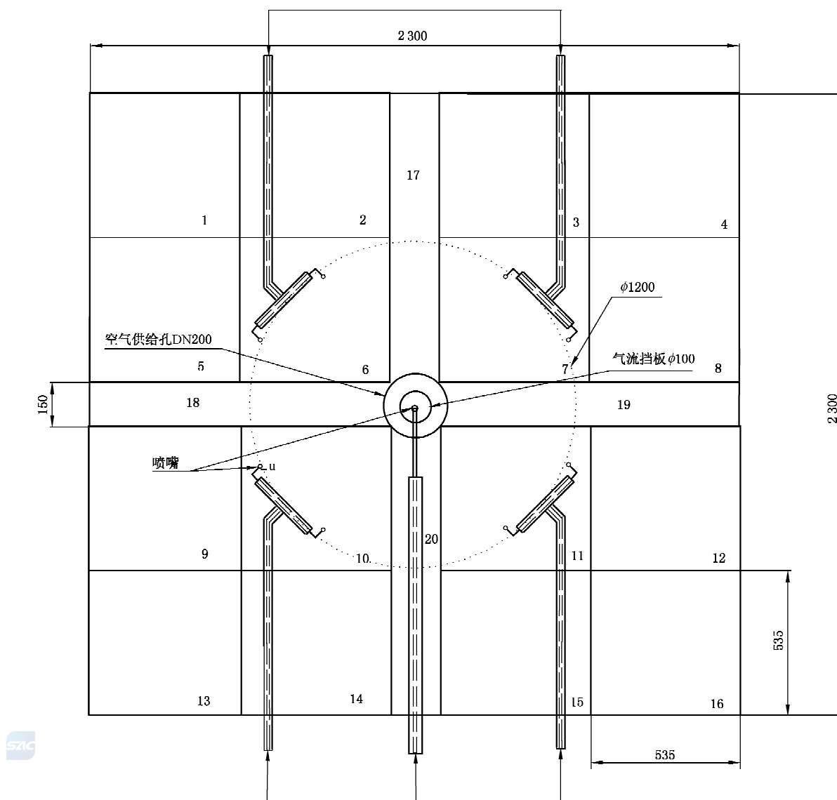
图 10 实际洒水密度(ADD)试验装置
