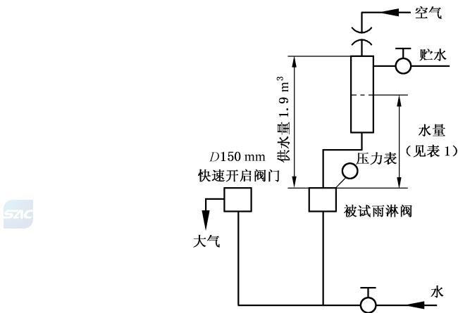
图 3 防复位试验
