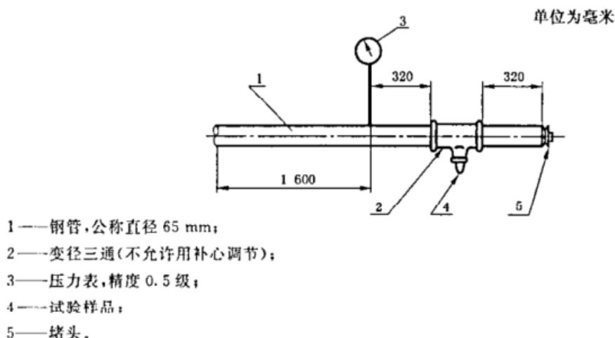
图 1 流量特性试验装置
