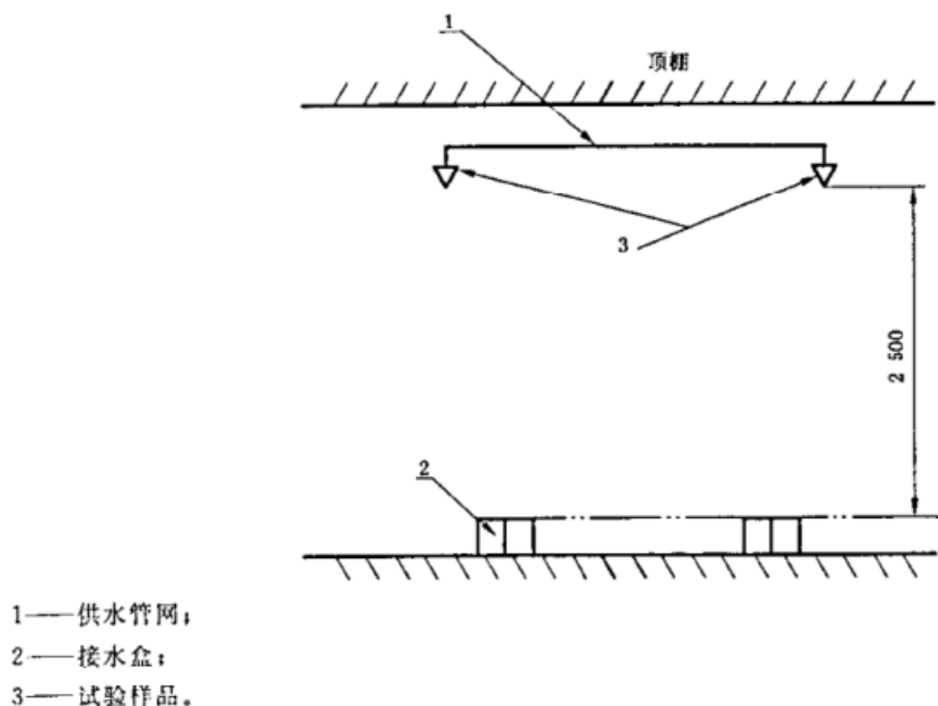
图4 洒水分布试验布置图
