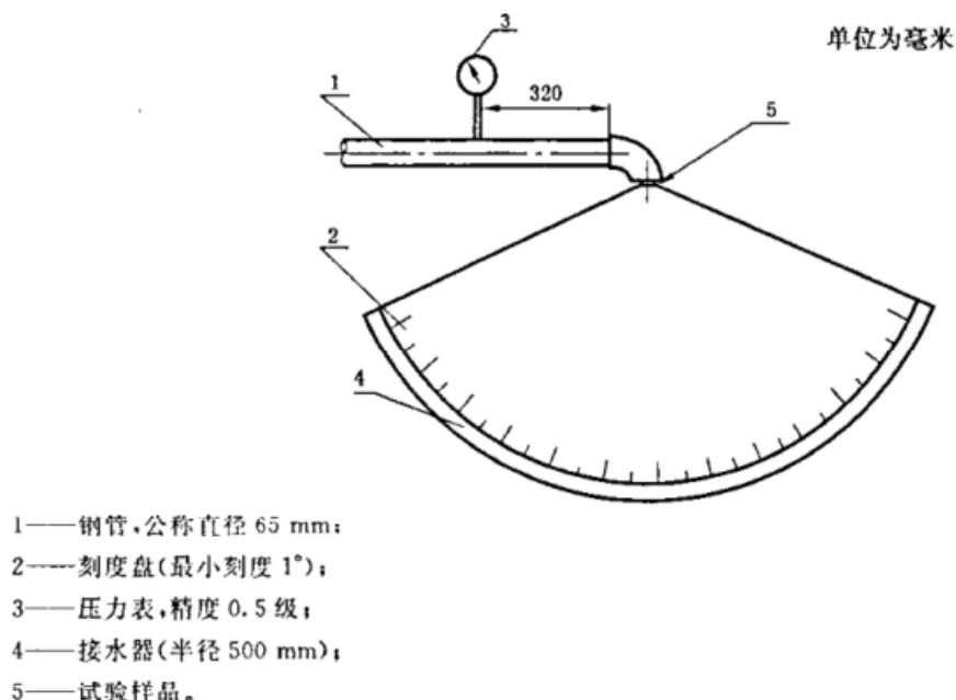
图 2 雾化角测试装置
