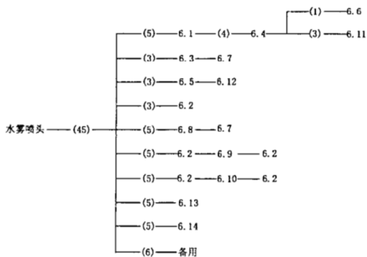
图 5 开式水雾喷头试验程序和样品数量
