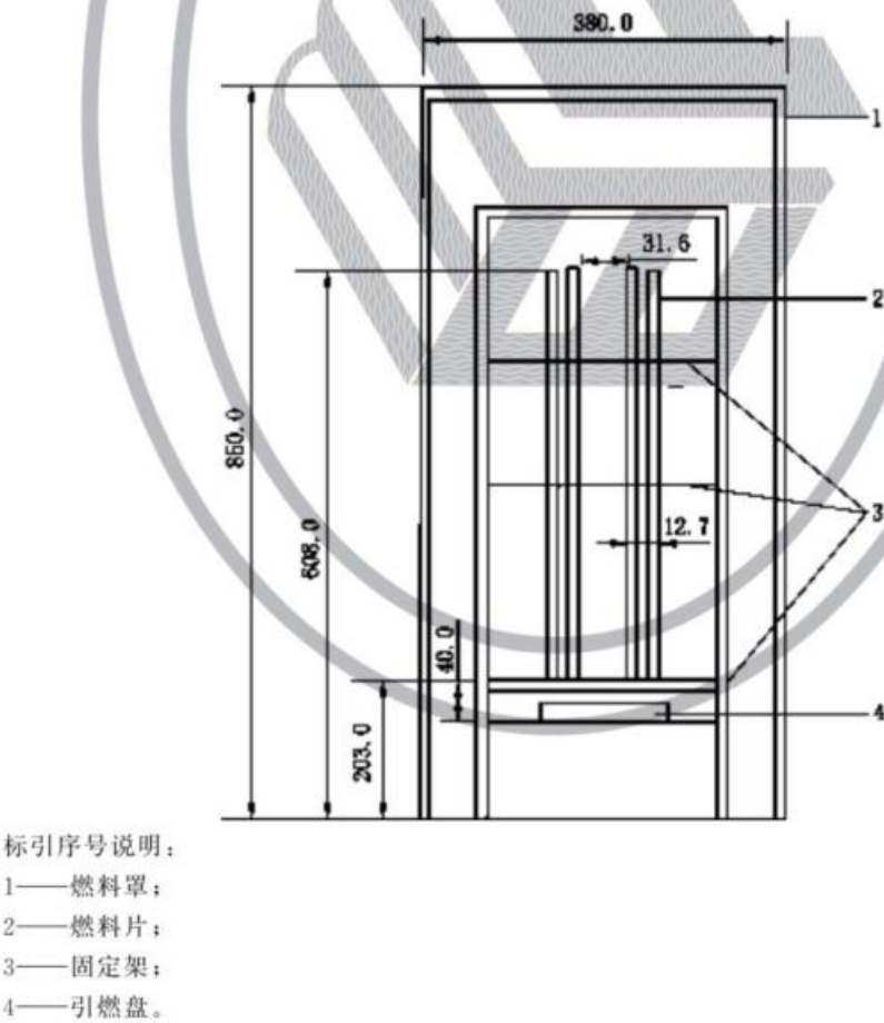
图 5 聚丙烯火试验模型示意图
