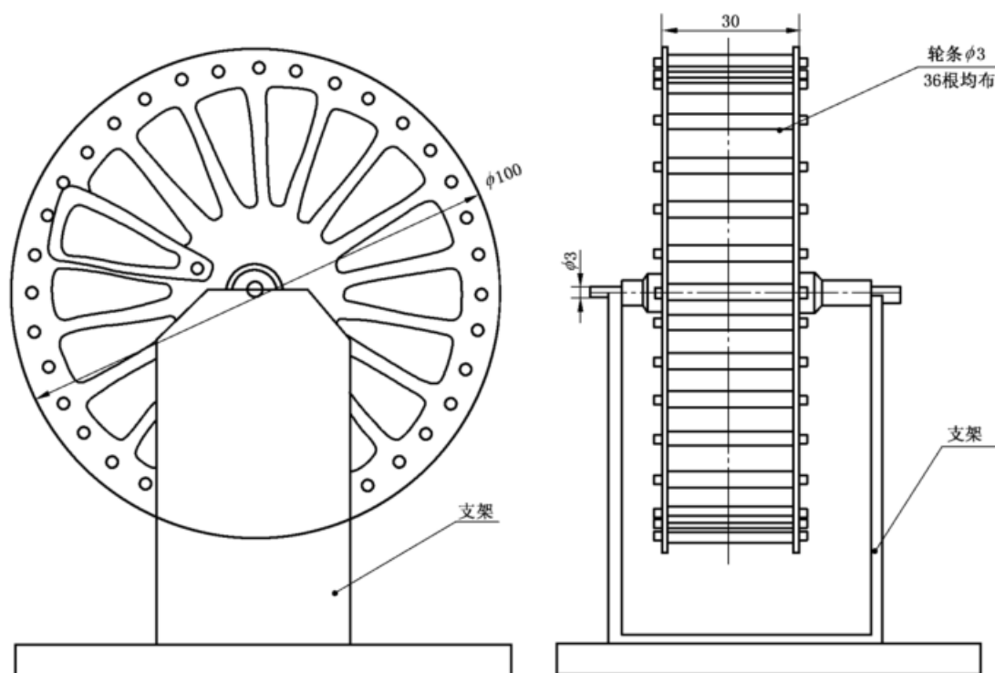
图3 小鼠转笼
