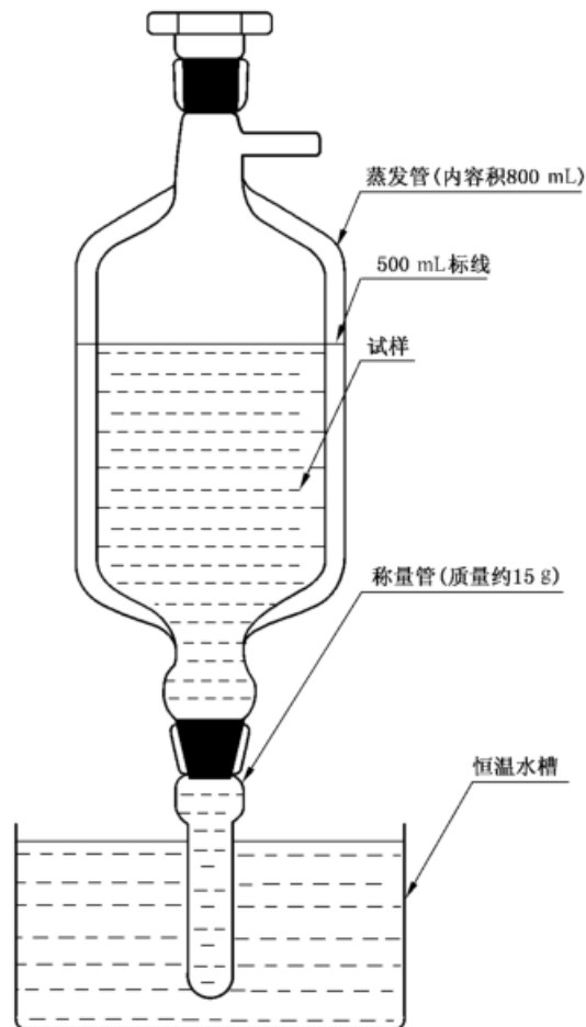
图 1 蒸发器
