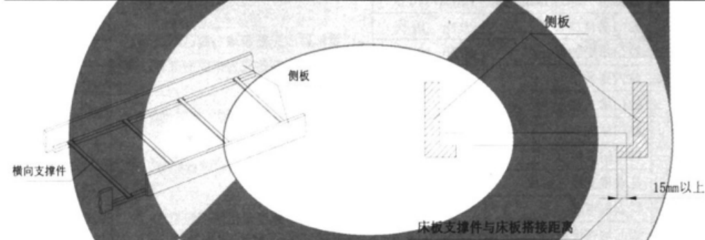
图 4 床板防落支撑件
